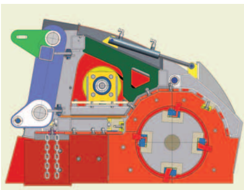
Μοντέλο σε τομή/ πλευρική άποψη του PTH crusher.
